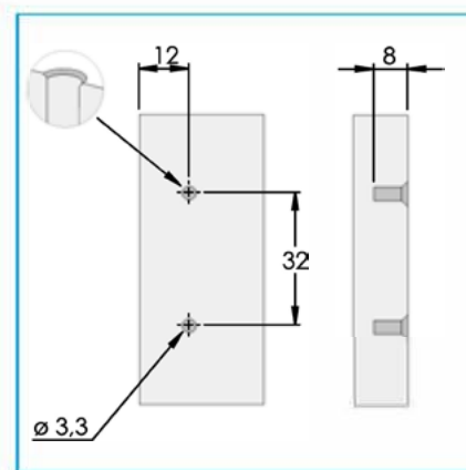
Bohrbild Seite
