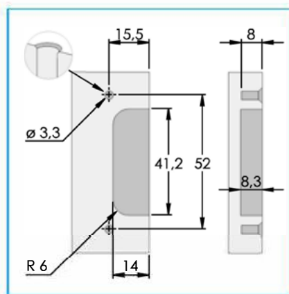
Bohrbild Tür
